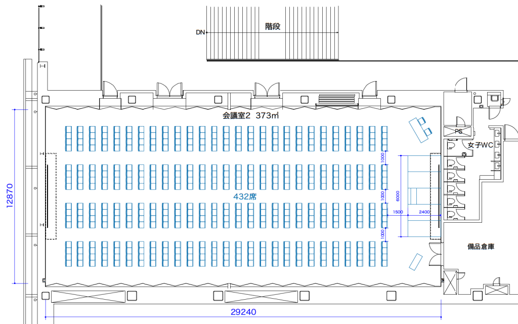
シアター形式レイアウト (1室利用)
