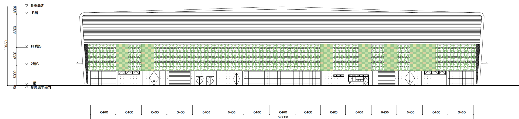
南側 立面図 S=1/400
