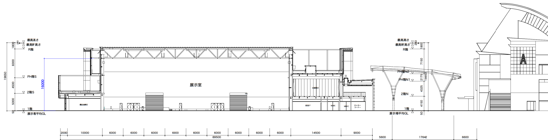
南北西寄断面図 S=1/400
