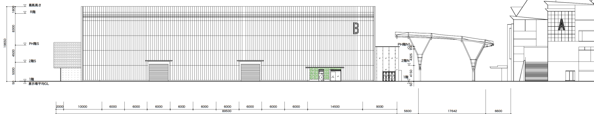
東側 立面図 S=1/400
