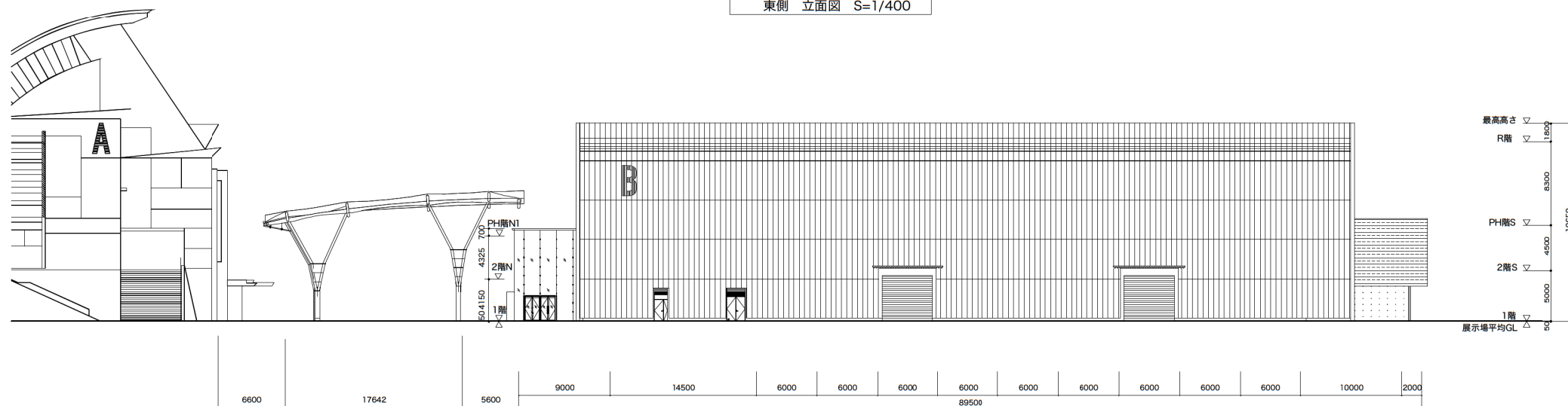
東側 立面図 S=1/400
