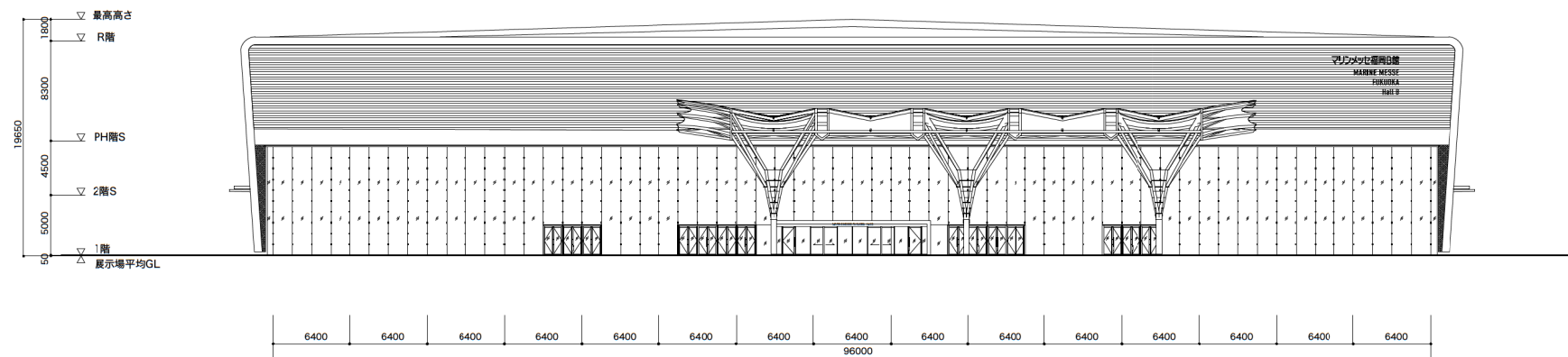
北側 立面図 S=1/400
