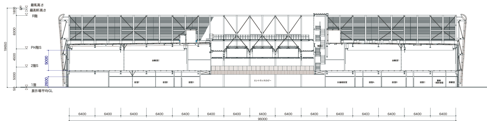
東西北側断面図 S=1/400
